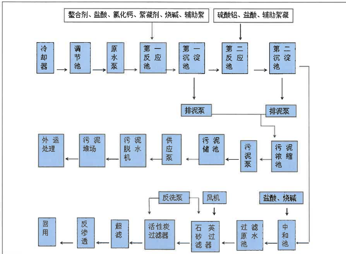
一期洗烟废水处理工艺
